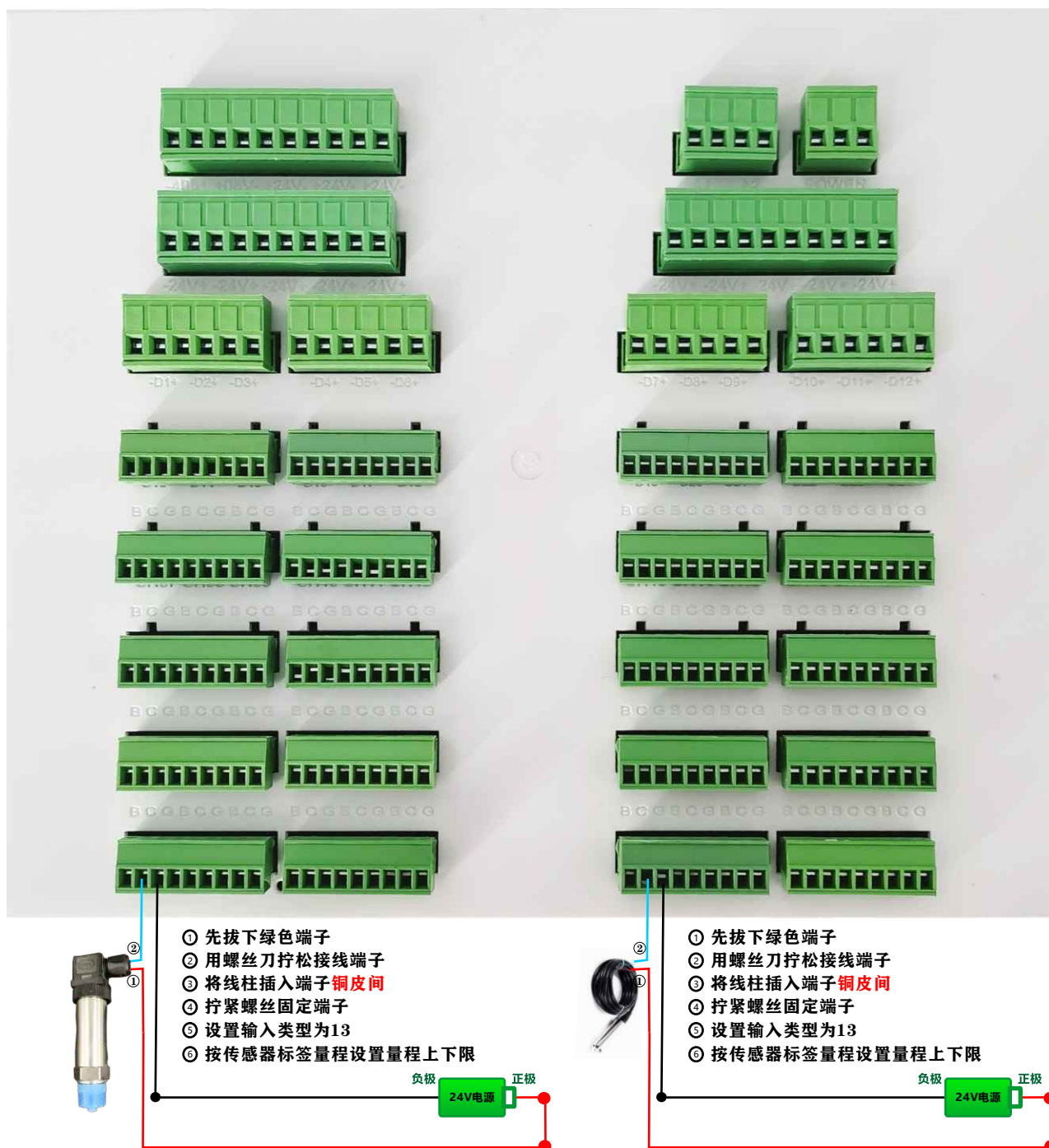
两线制压力变送器接线
