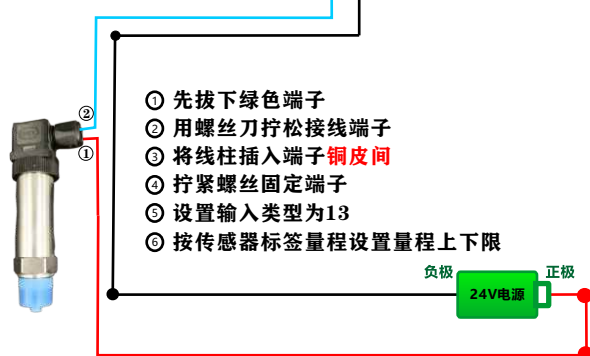
两线制压力变送器接线
