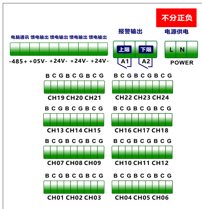
不带控制仪表接线
