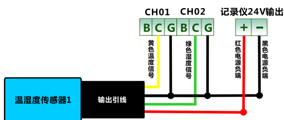
温湿度接线图
