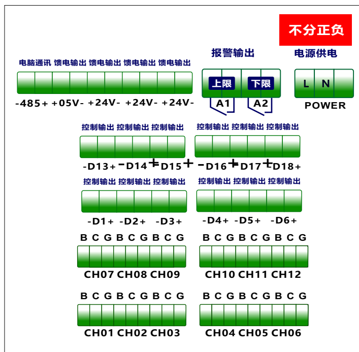
带控制仪表接线
