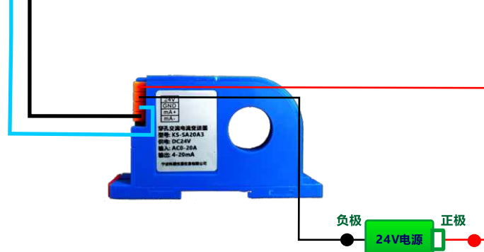
适用于四线制供电型变送器
