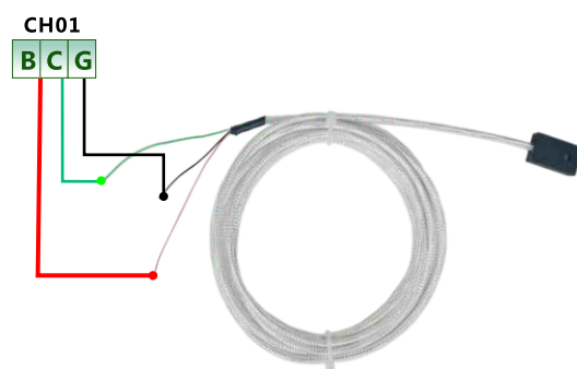
湿度传感器接线
